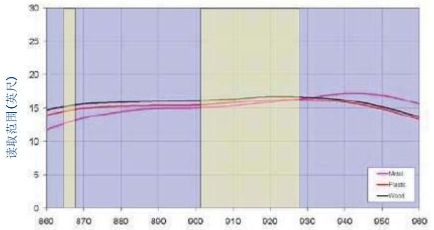
“小型Gen2耐用标签”的读取范围性能
